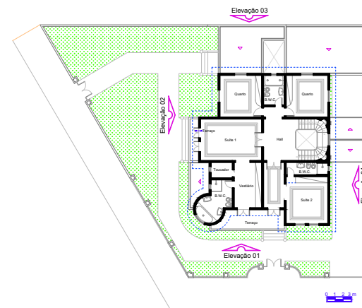
Superior
