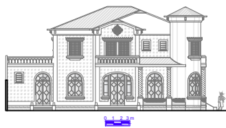
Elevação 02
