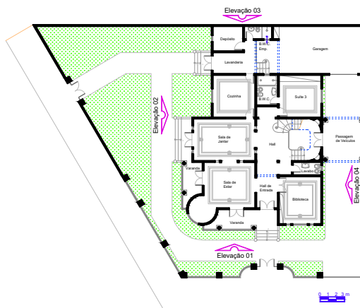
Térreo
